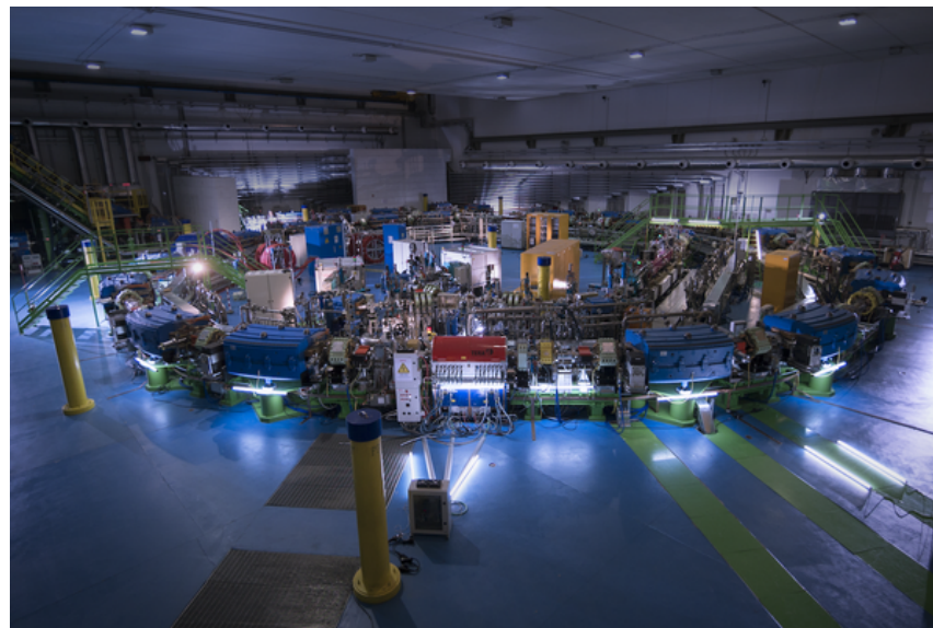
L'acceleratore di particelle del CNAO
